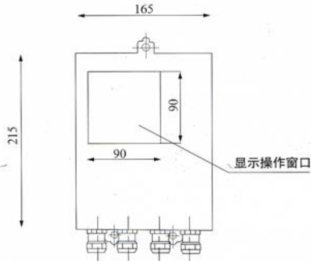
转换器外观尺寸 165×215×70(宽高厚)
