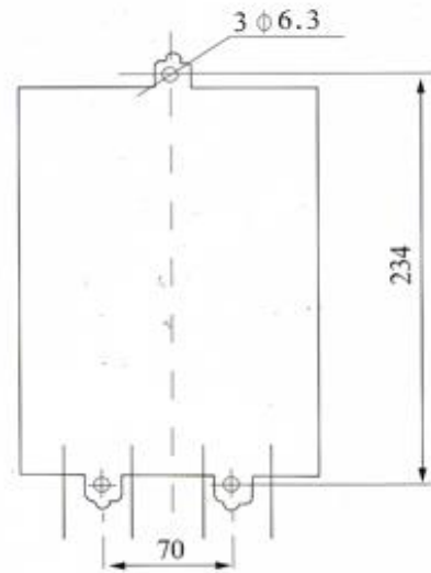
转换器安装尺寸(墙壁挂式)
